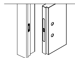
Serratura magnetica con foro nottolino WC
