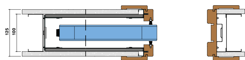
SPESSORE CONTROTELAIO 125 Lastra singola
