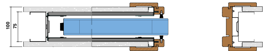
SPESSORE CONTROTELAIO 100 Lastra singola
