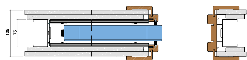
SPESSORE CONTROTELAIO 100 Lastra doppia
