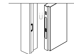
Magnetic strike plate – Touch with SLIM pull handle / Gâche magnétique – Touch avec poignée SLIM
