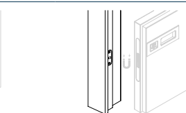
Kit Maniglia Adapta con nottolino
