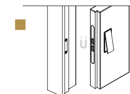
Incontro magnetico Touch con leva tira porta a incasso LARGE
