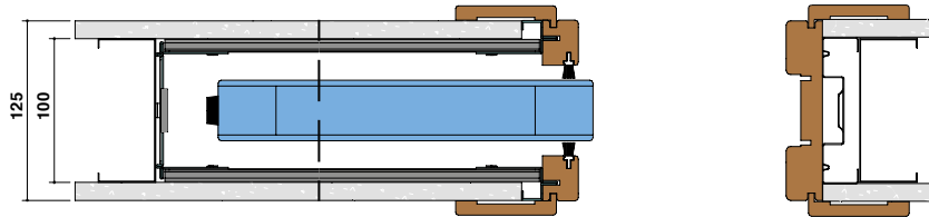
SPESSORE CONTROTELAIO 125 Lastra singola
