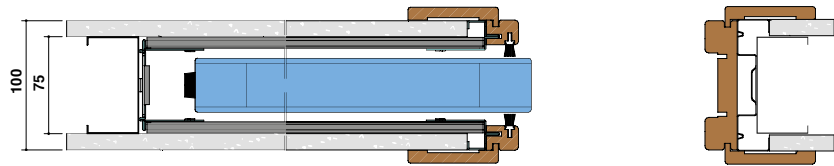
SPESSORE CONTROTELAIO 100 Lastra singola
