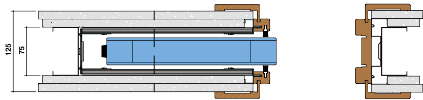
SPESSORE CONTROTELAIO 100 Lastra doppia
