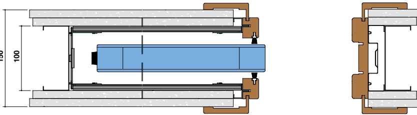
SPESSORE CONTROTELAIO 125 Lastra doppia
